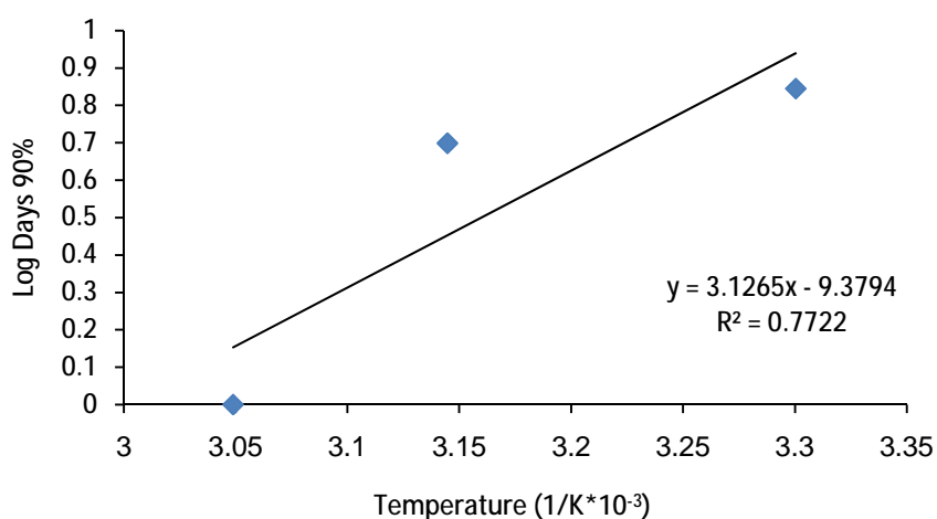
نمودار 6: لگاریتم 90% t در برابر عکس دمای مطلق در مورد ژل 0/2 درصد ایندومتاسین تهیه شده با HPC 5 درصد
