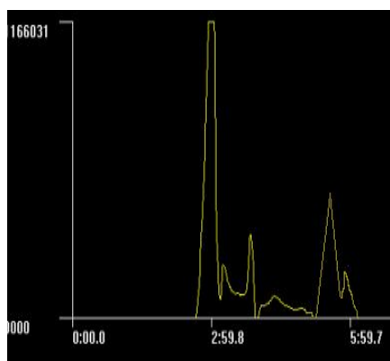
شکل 2- کروماتوگرام بدست آمده برای ان-استیل سیستین استاندارد با غلظت 50µg/ml
