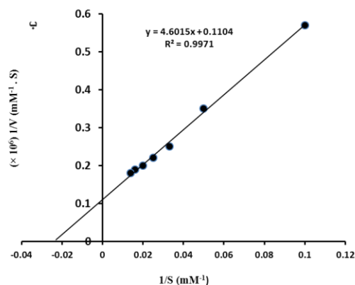
شکل ۱. الف) نمودار میکائیلیس - منتن آنزیم کاتالاز کبد گاو در دمای ۲۵ درجه سانتی‌گراد ب) نمودار لاینیوبریک برای آنزیم کاتالاز کبد گاو در دمای ۲۵ درجه سانتی‌گراد.
