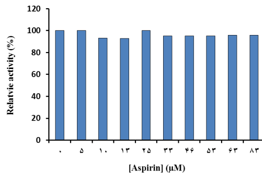
شکل ۲. درصد فعالیت نسبی کاتالاز تحت تاثیر غلظت‌های مختلف آسپیرین در دمای محیط
