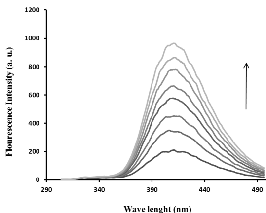
شکل ۵. شدت نشر فلئورسانس غلظت‌های مختلف آسپیرین (از پایین به بالا (از پایین به بالا ۰، ۲، ۴، ۶، ۸، ۱۰، ۱۲، ۱۴ و ۱۶ میکرو مولار) در دمای ۲۵ درجه ی سانتیگراد.
