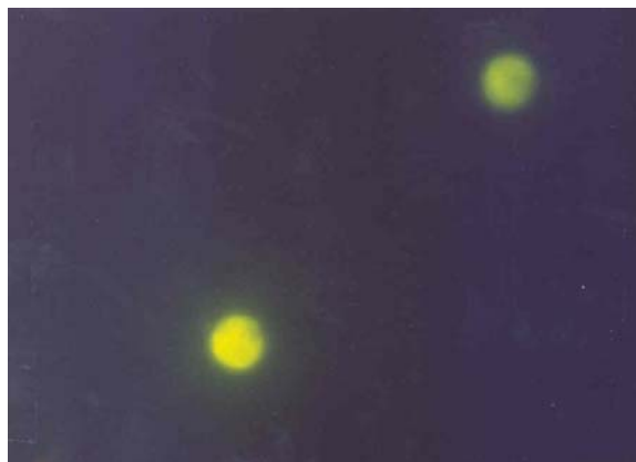
شکل ۲. رنگ آمیزی نمونه بیمار به روش فلئوئورسانس با ردامین. بزرگ نمایی: \times 1000
