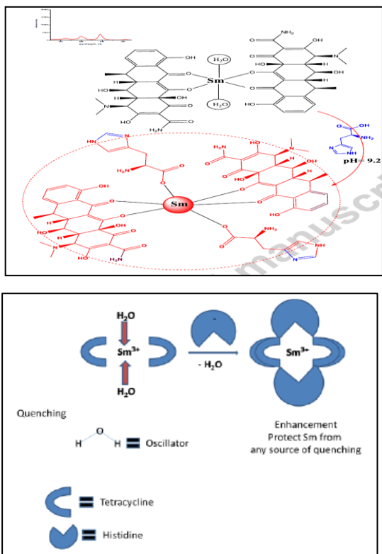
شکل (۸) مکانیسم واکنش هیستیدین با نانوپروپ نوری ساماریوم-تتراسایکلین (بالا)، محافظت از یون ساماریوم در برابر خاموش کننده (پائین) [۴۰].
