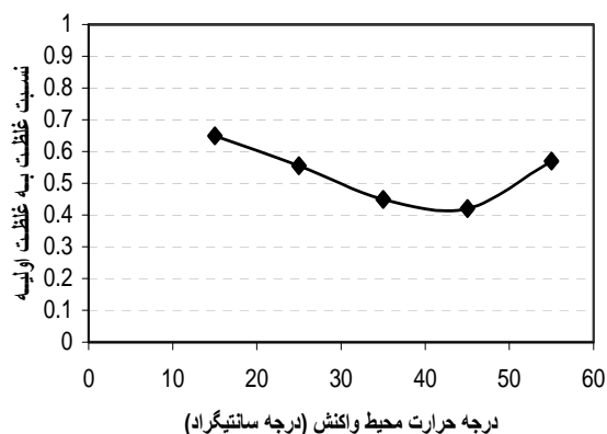
شکل ۴- تأثیر درجه حرارت بر جذب رنگ (راکتیو قرمز ۱۳۳)
