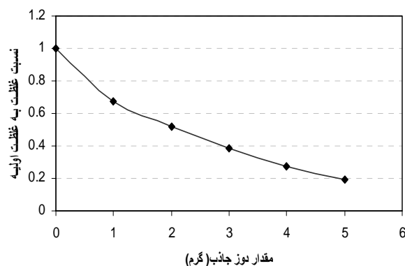
شکل ۵- تأثیر دوز جاذب در حذف رنگ راکتیو قرمز ۱۳۳
