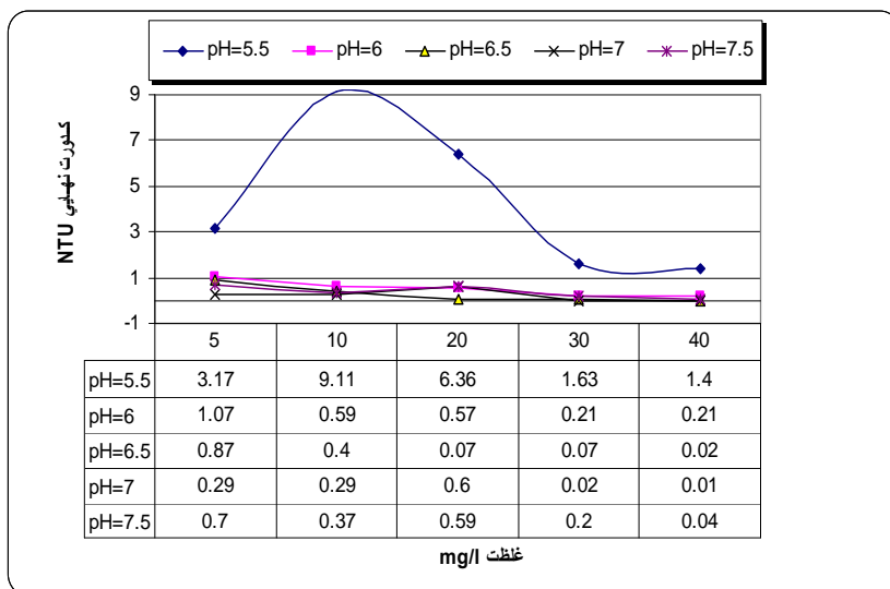
نمودار شماره ۴- کدورت نهایی در غلظت ها و pH های مختلف منعقد کننده کلراید فریک با کدورت اولیه ۱۳.۹ NTU
